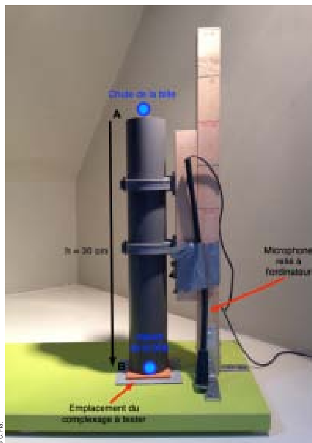
Figure 1. Montage expérimental.
